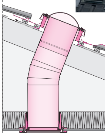
Сечение Туннеля дневного света SRD
