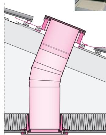
Сечение Туннеля дневного света SR_
