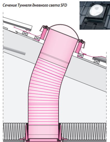
Сечение Туннеля дневного света SFD
