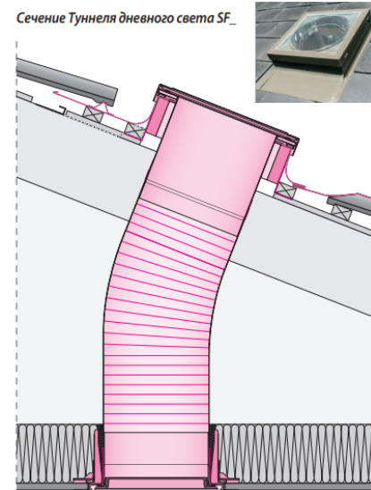
Сечение Туннеля дневного света SF_
